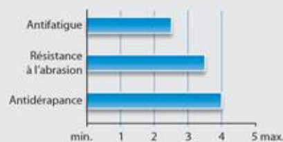
Brosses + jonctions
